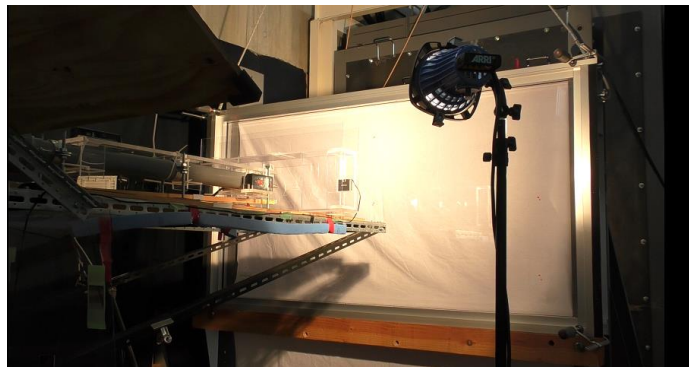
写真1 アルミ枠付き遮音板の衝撃試験の様子
